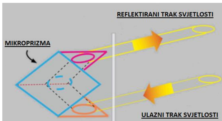
Slika 12. Prizmatična retrorefleksija
