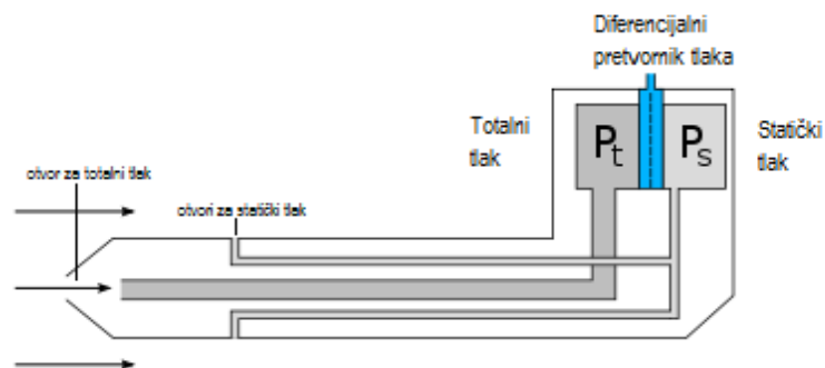
Slika 4. Pitot-statička cijev
