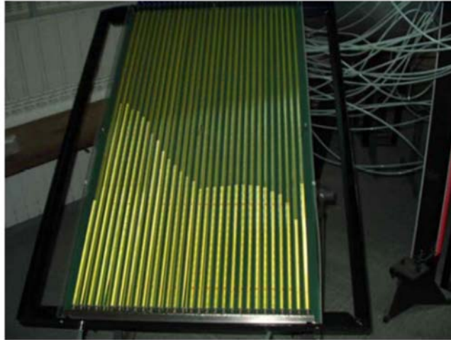
Slika 40. Piezometarska harfa
