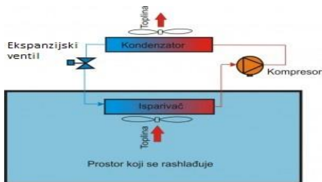
Slika 18. Osnovna shema najjednostavnijeg rashladnog pogona
