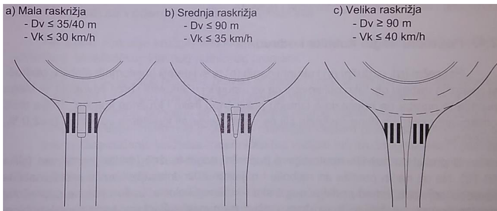
Slika 20. Oblici razdjelnih otoka u zavisnosti o veličini (Dv) i brzini uvoženja (Vk); (a) paralelni; (b) trokutasti i (c) ljevkasti
