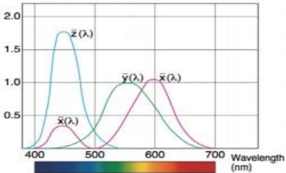
Slika 4. - Grafički prikaz funkcija, CIE 1931.
