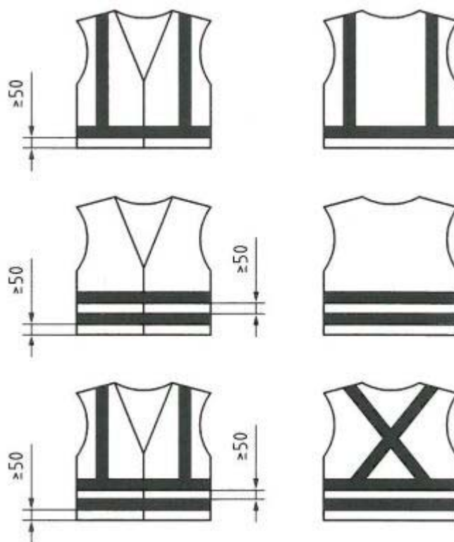
Slika 3. Primjer odjeće visoke vidljivosti koja pokriva torzo (mjere u milimetrima).
