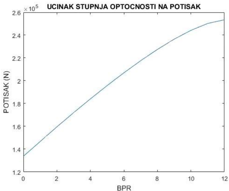
Slika 12. Utjecaj povećanja stupnja optočnosti na potisak
