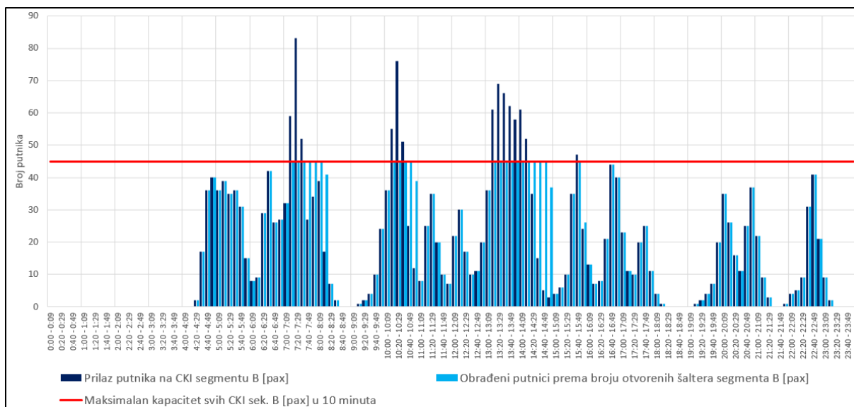
Grafikon 73. Prikaz maksimalnog kapaciteta segmenta „B“ u odnosu na stvarni priljev i realnu obradu putnika tijekom tipičnog poslovnog dana (15. 8. 2014.) Izvor: Izradio autor prema bazi podataka Zračne luke Zagreb iz 2014. godine
