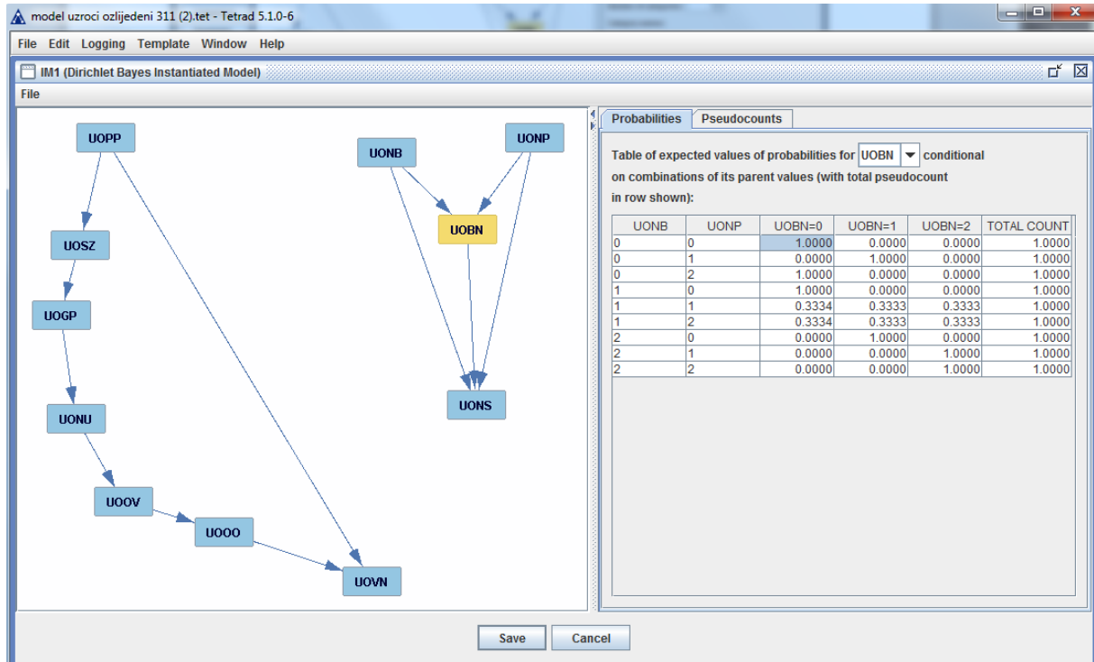
Slika 6. Bayesov model djelovanja – Model 2
