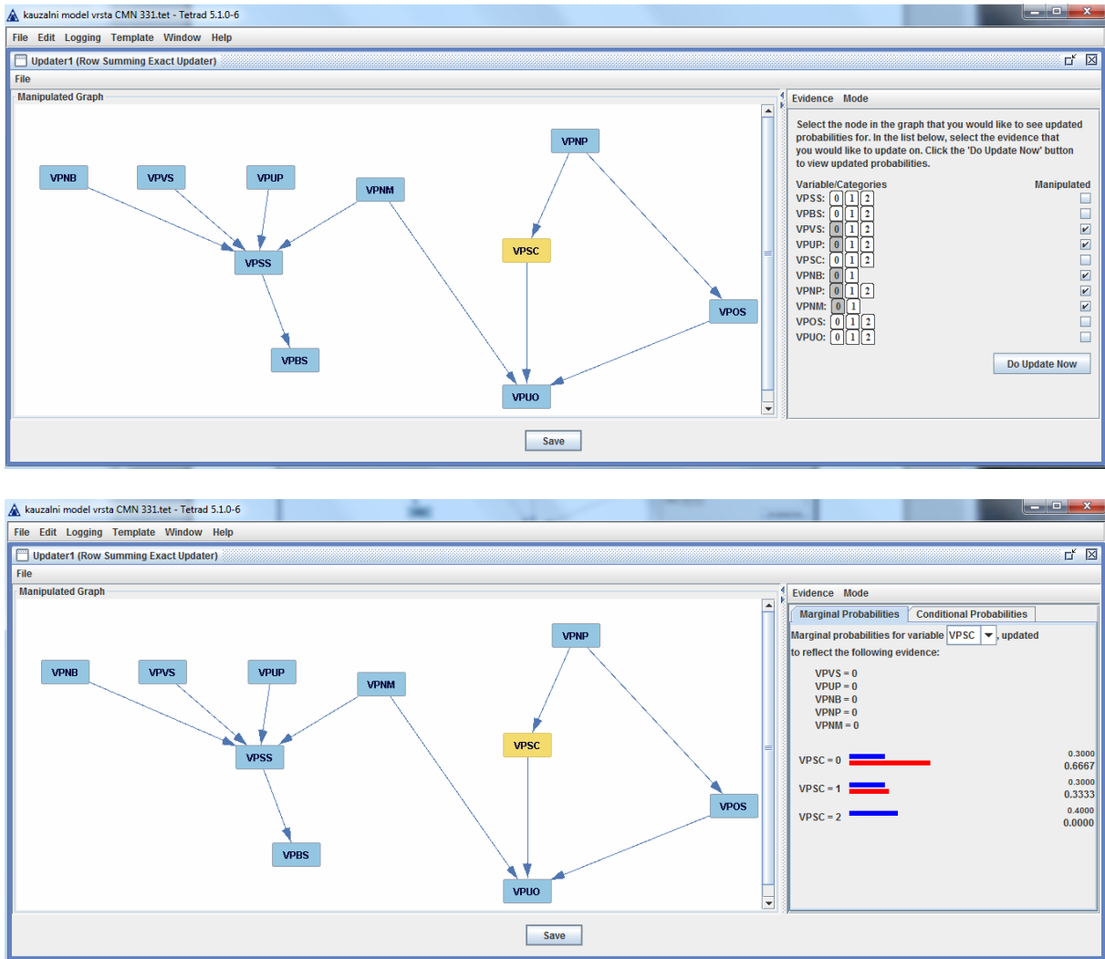
Slika 7. Grafički prikazi provedbe simulacije modela – Model 3
