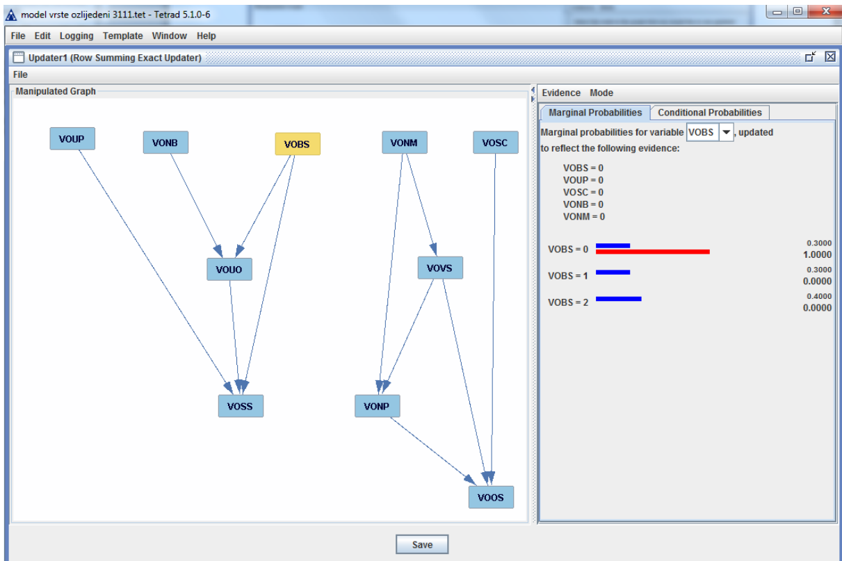
Slika 7. Grafički prikazi provedbe simulacije modela – Model 4
