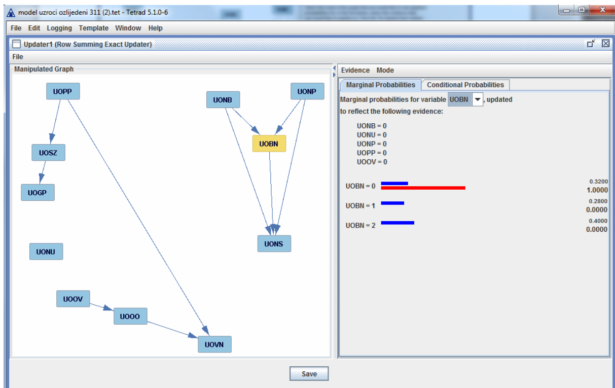
Slika 7. Grafički prikazi provedbe simulacije modela – Model 2
