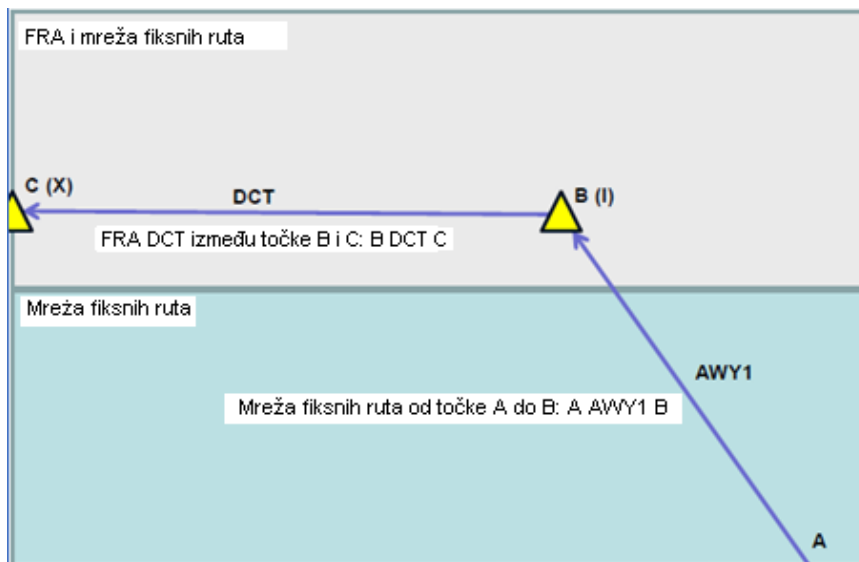
Slika 5. Putanja zrakoplova u odlasku, iz prostora mreže fiksnih ruta u FRA prostor [3]
