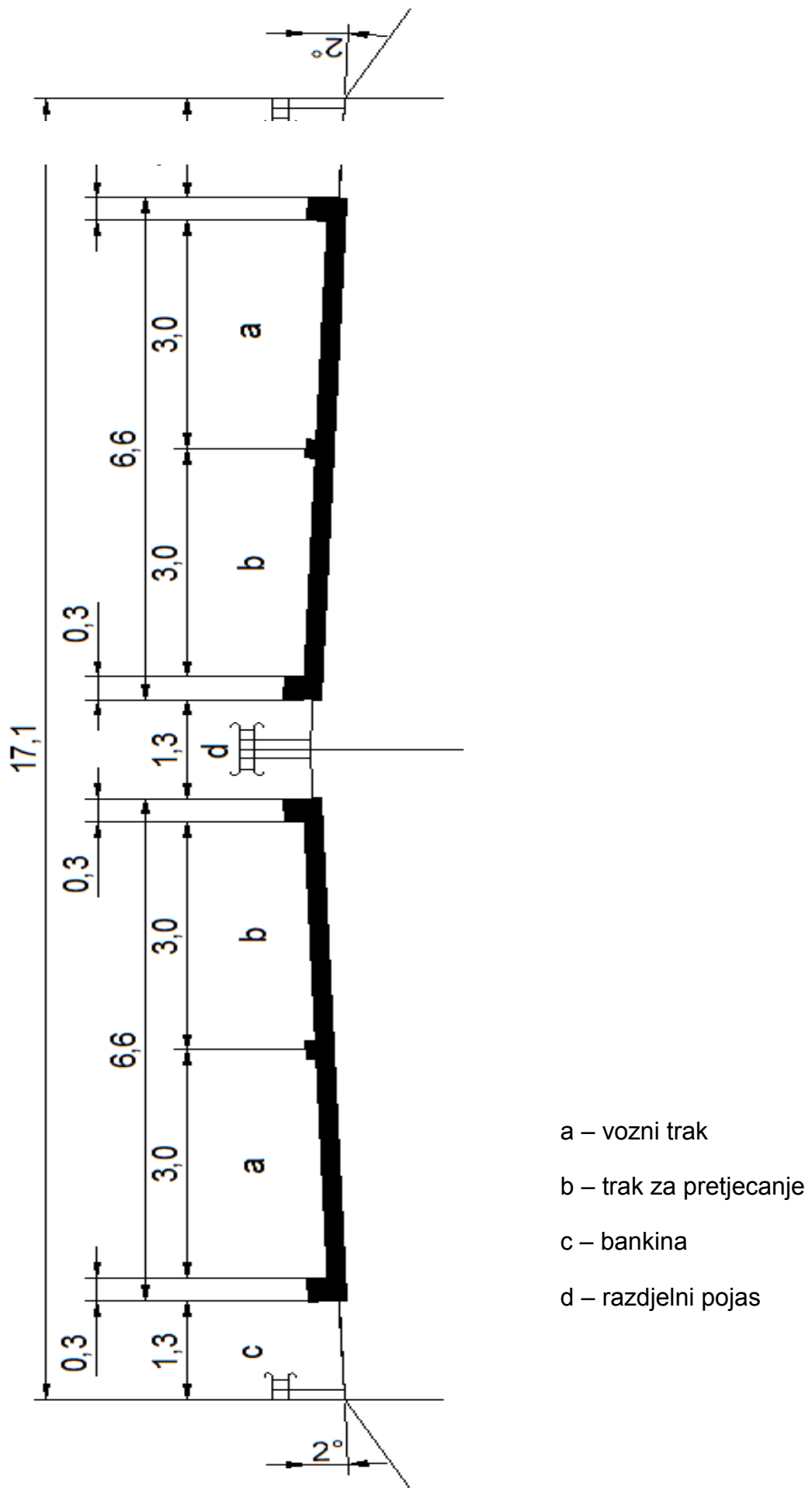
Slika 20.: Poprečni profil ceste za premoščavanje, V_{pl} = 70, 60 km/h (izradila autorica)
