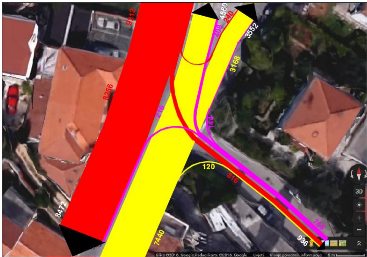
Slika 27. Dnevno opterećenje prometnih tokova na raskrižju 3 u kolovozu Izvor: [52]
