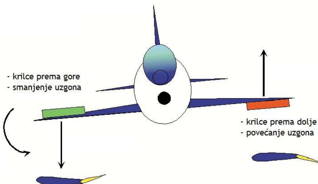
Slika 19. Utjecaj krilaca
