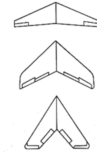
Slika 7. Veliki i mali kut strijele
