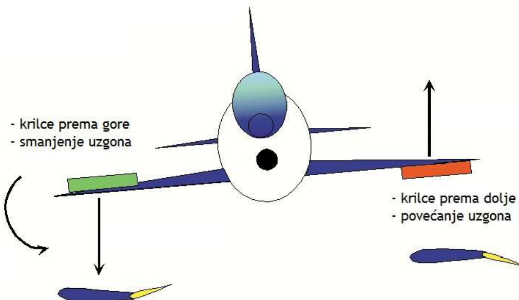
Slika 19. Utjecaj krilaca
