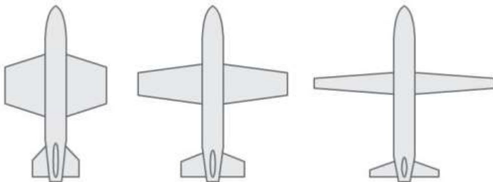
Slika 16. Vitkost krila
