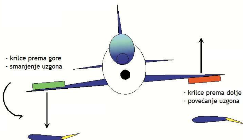
Slika 19. Utjecaj krilaca
