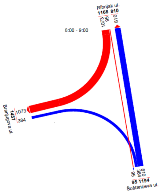
Slika 7. Grafički prikaz prometnih tokova kroz karakteristično raskrižje Šoštarićeve – Branjugove – Ribnjak ulice (Langov trg) u vremenu od 8:00 do 9:00h
