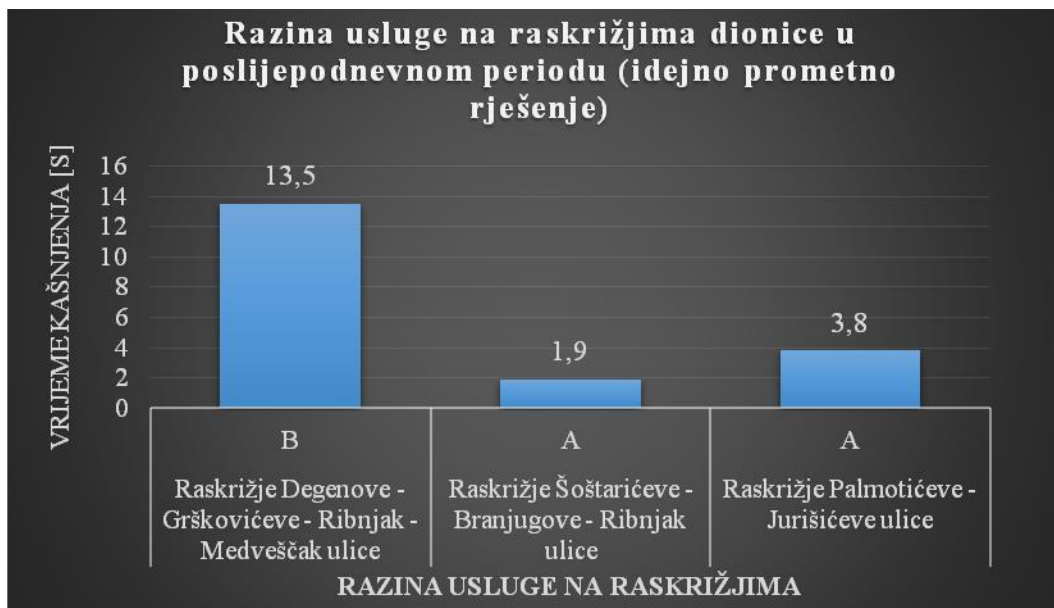
Grafikon 13. Razina usluge na raskrižjima u poslijepodnevnom periodu – idejno prometno rješenje
