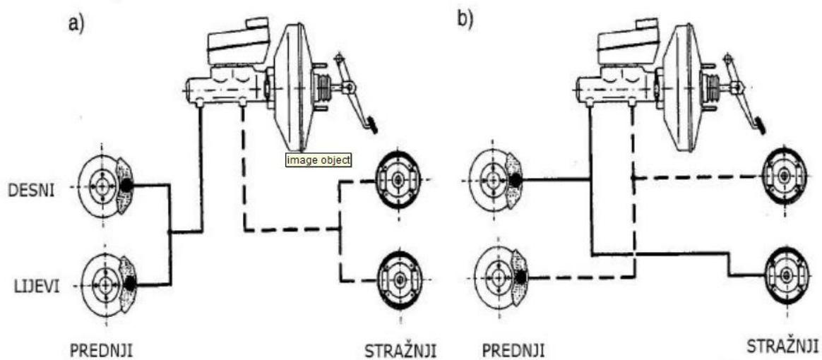
Slika 5. Podjela kočnih krugova
