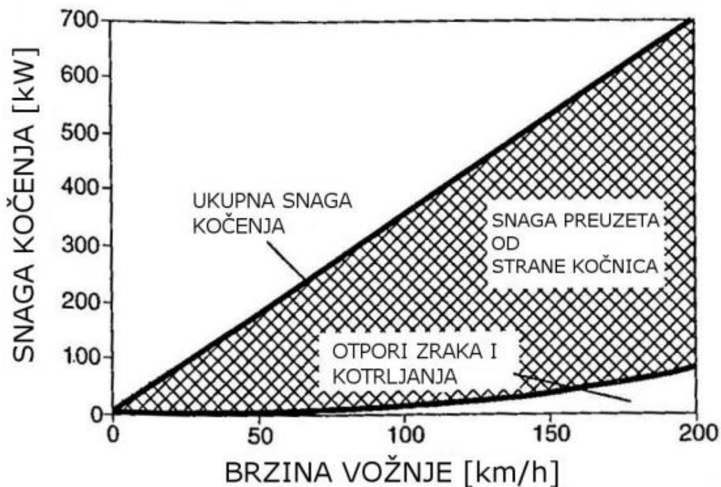
Slika 7. Prikaz omjera snage kočenja s obzirom na brzinu vožnje pri usporencu 1G
