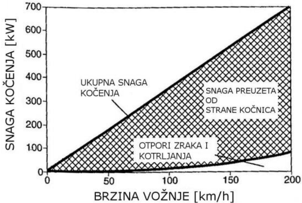
Slika 7. Prikaz omjera snage kočenja s obzirom na brzinu vožnje pri usporenu 1G
