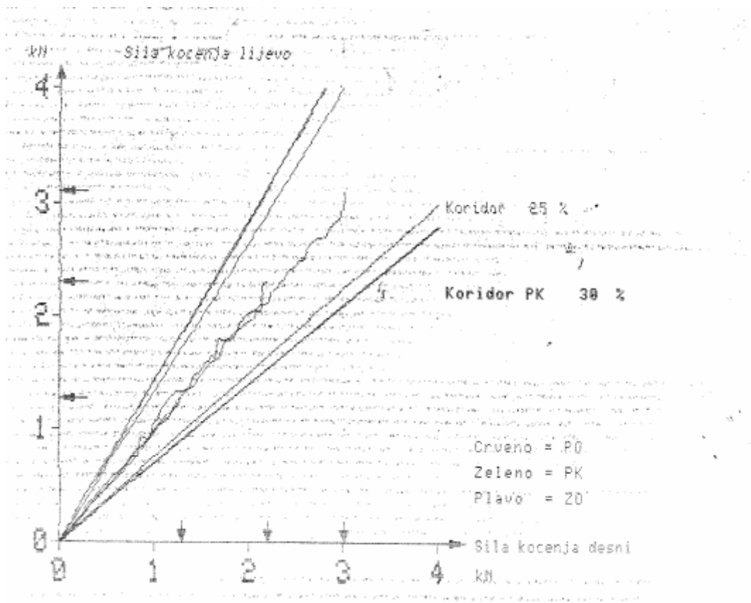
Slika 10. Prikaz dijagrama ispitivanja kočnica
