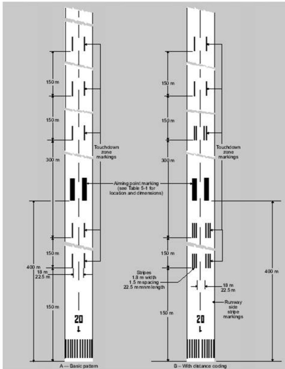
Slika 4. Oznake područja dodira, ruba i ciljne točke
