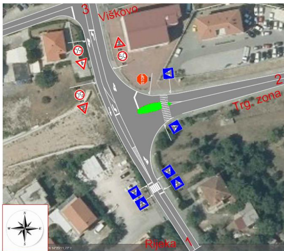
Slika 11. Tlocrtni prikaz raskrižja
