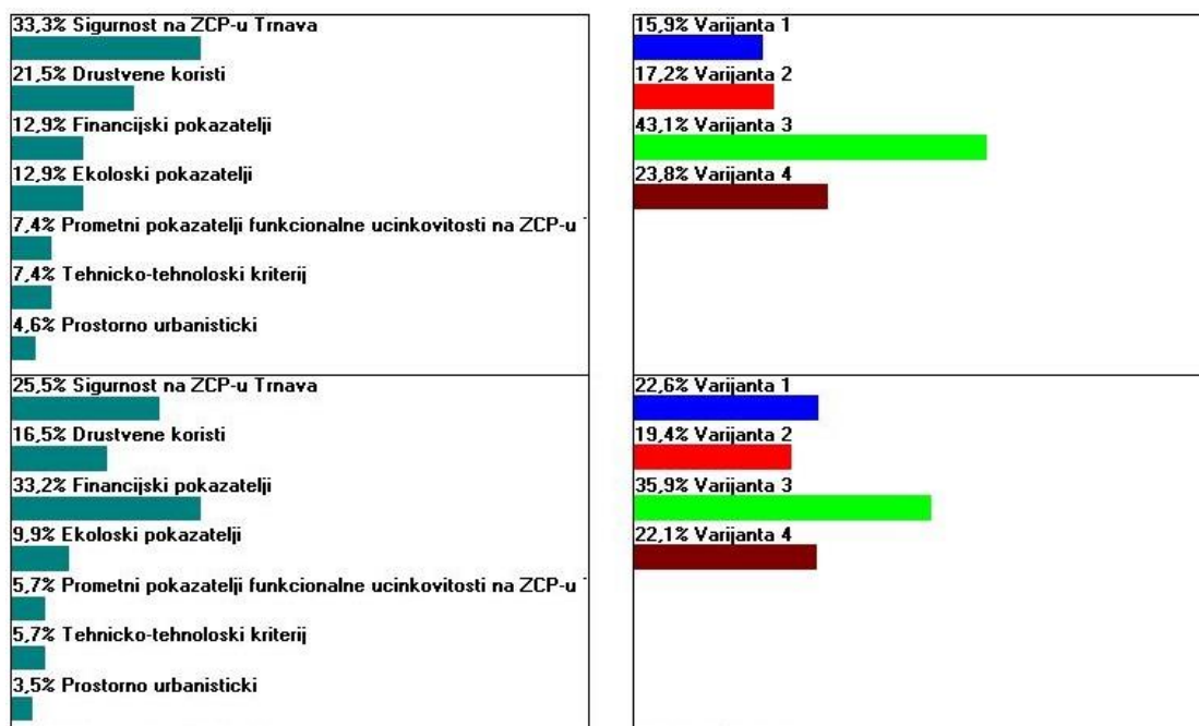
Slika 67. Analiza osjetljivosti
