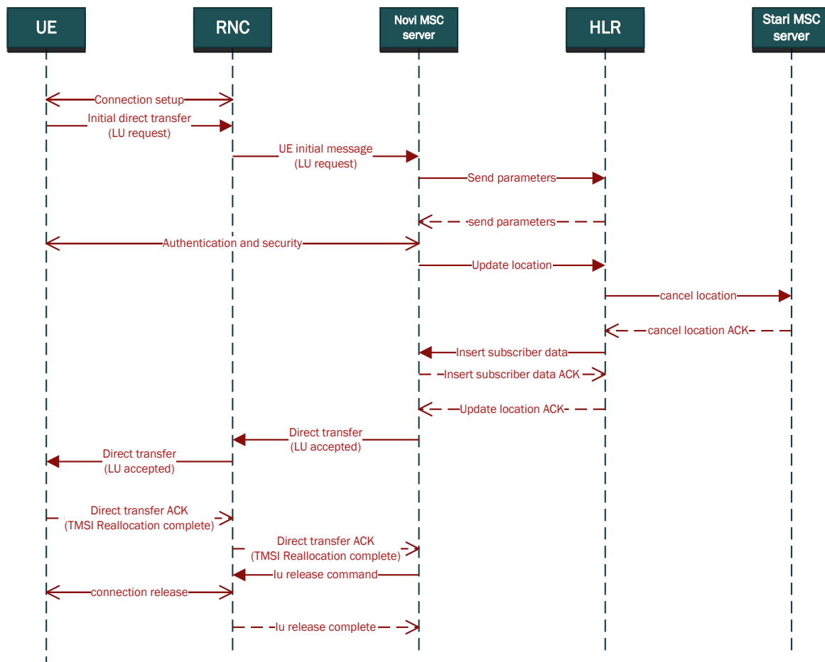
Slika 7: Proces ažuriranja lokacije Izvor: [5]
