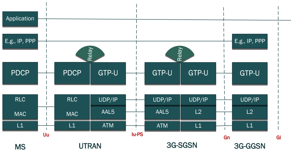
Slika 4: Protokolarni složaj za korisničku ravninu Izvor: [10]
