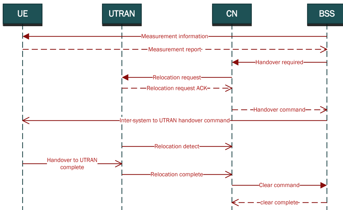
Slika 14: Prekapćanje sa GSM na UTRAN mrežu Izvor: [15]
