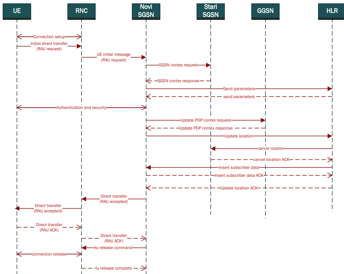
Slika 8: RAU proces Izvor: [5]
