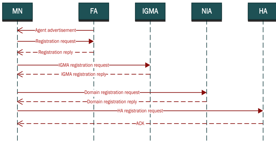
Slika 21: Tijek signalizacije prilikom prekapčanja izvan domene Izvor: [19]
