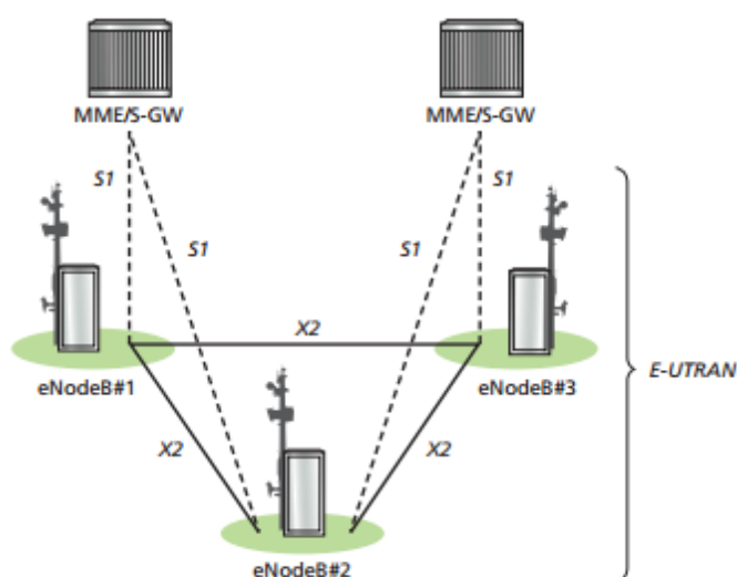
Slika 15. E-UTRAN mrežna arhitektura, [14]
