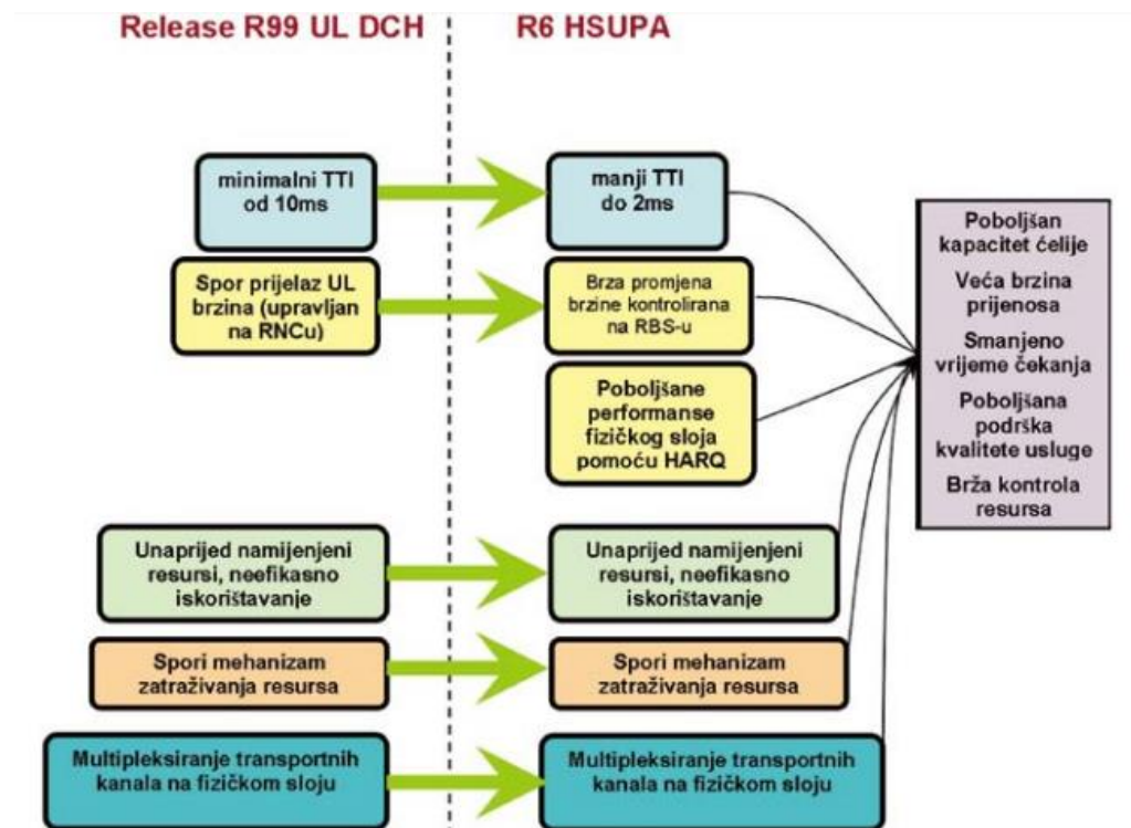
Slika 8. Usporedba funkcionalnosti sustava prema R99 i HSUPA tehnologije prema R6, [15]
