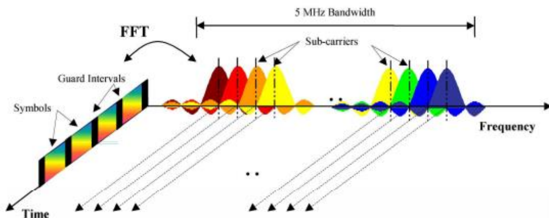
Slika 10. Prikaz OFDM modulacijske tehnike, [12]
