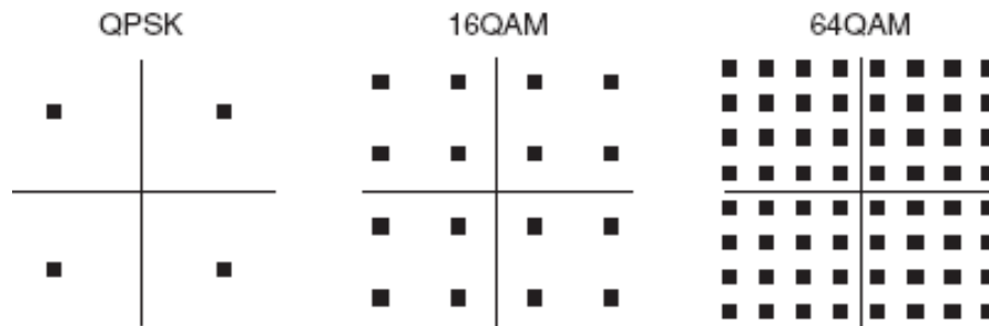
Slika 7. QPSK, 16 QAM i 64 QAM dijagrami stanja, [5]
