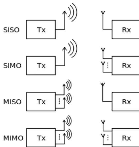
Slika 11. Moguće kombinacije antenskih sustava s više ulaza i izlaza, [25]
