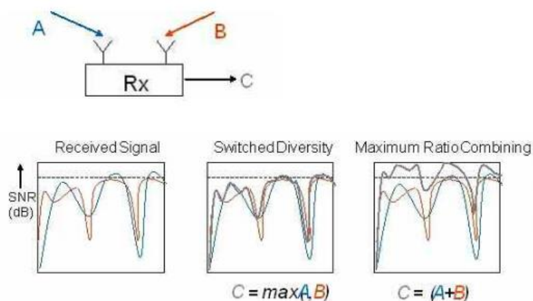
Slika 12. RX diversity, [22]
