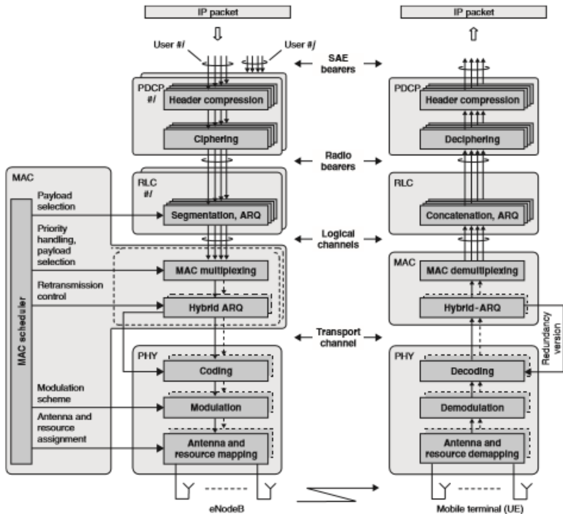
Slika 17. LTE protokolska arhitektura ( downlink ), [1]
