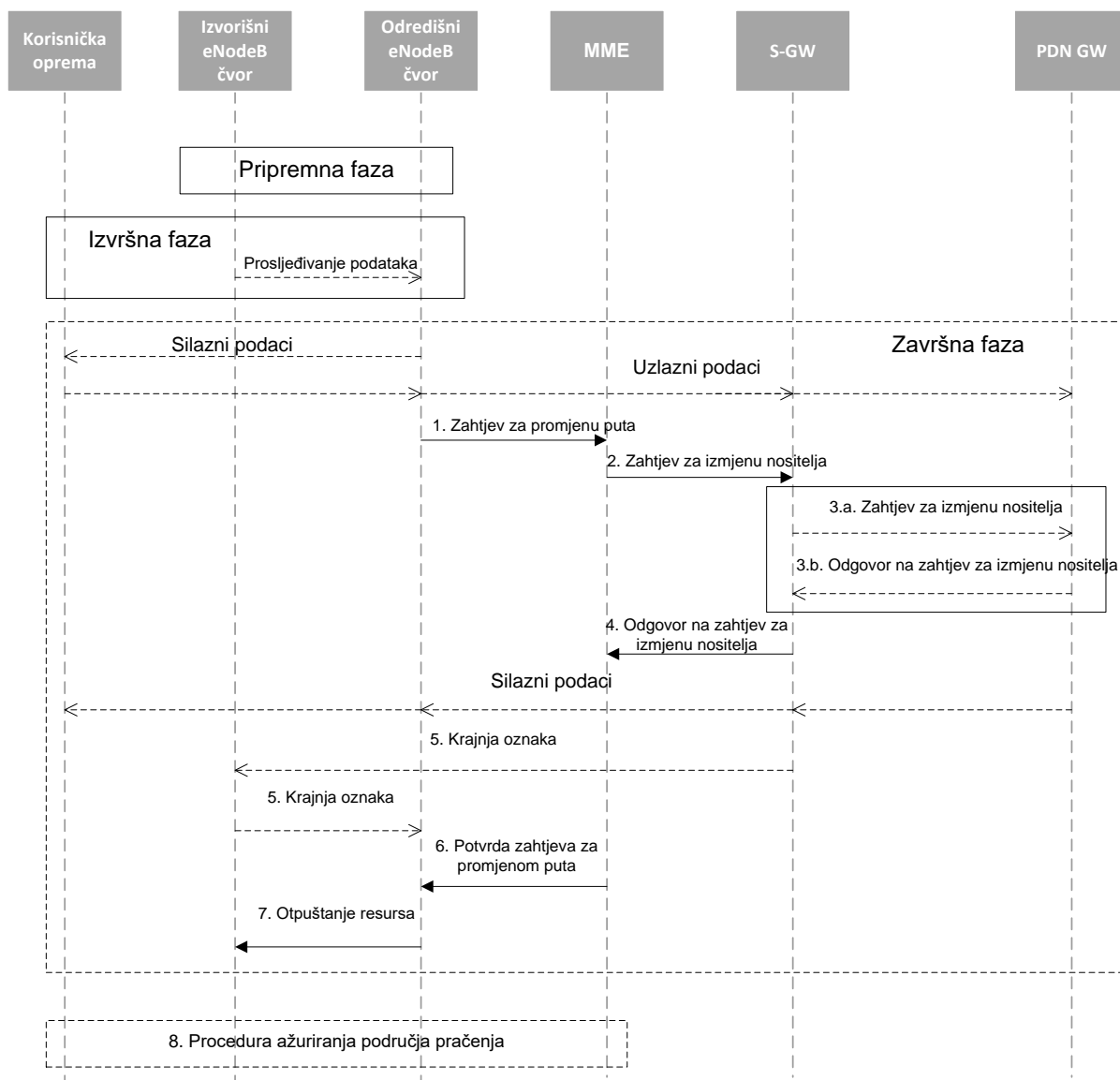
Dijagram 1. Intra LTE proces preuzimanja poziva bez promjene S-GW-a baziran na X2 sučelju, [23]
