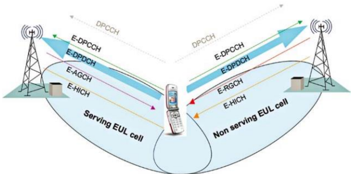
Slika 9. Konfiguracija HSUPA kanala, [15]
