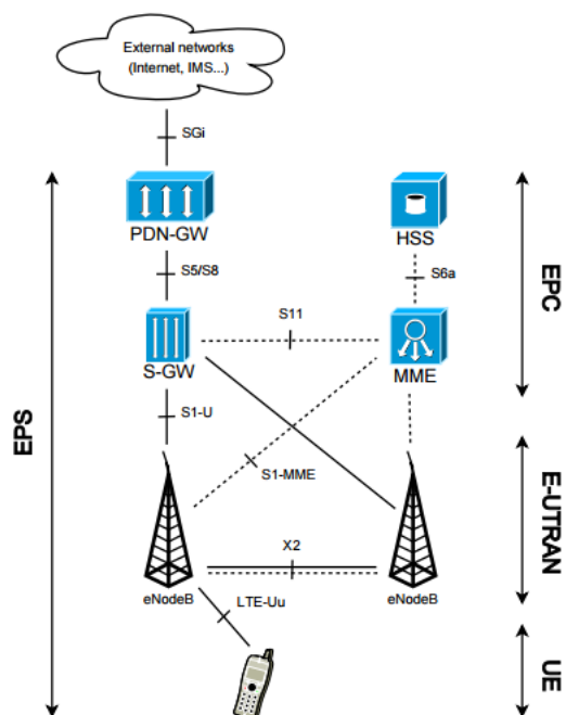
Slika 14. Mrežna EPS arhitektura, [11]
