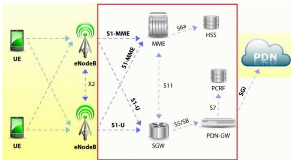
Slika 16. EPC mrežna arhitektura, [18]
