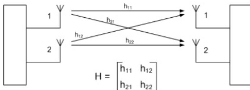
Slika 13. Konfiguracija MIMO 2x2, [22]
