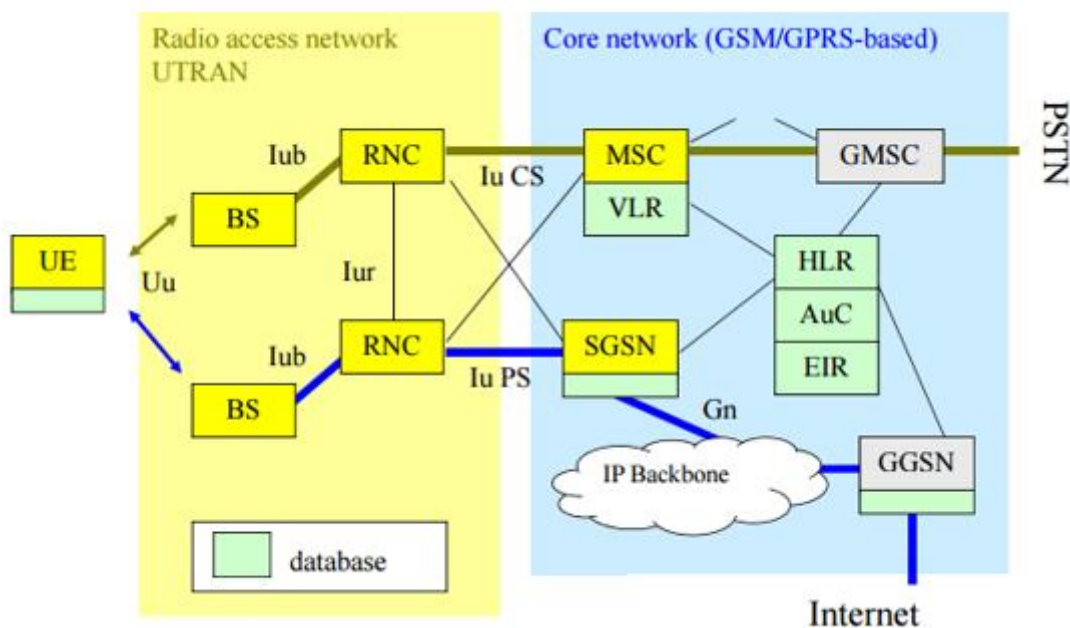
Slika 2. Mrežna arhitektura UMTS sustava, release 99 , [8]
