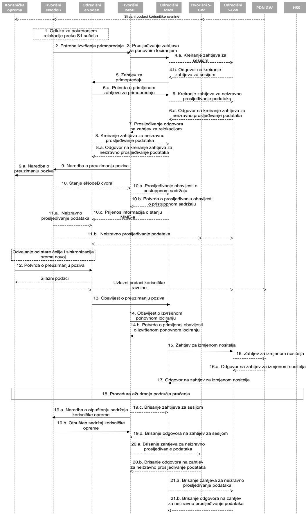
Dijagram 2. Intra LTE proces preuzimanja poziva baziran na S1 sučelju, [23]
