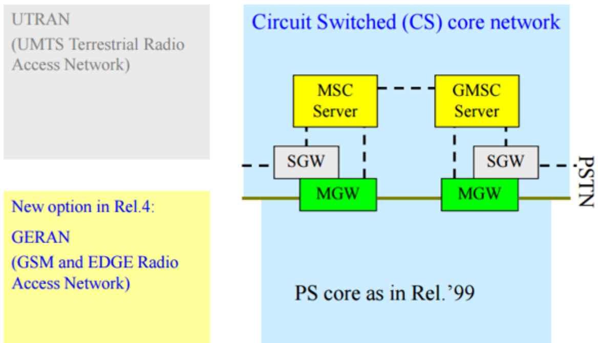
Slika 3. Mrežna arhitektura UMTS sustava, release 4 , [8]
