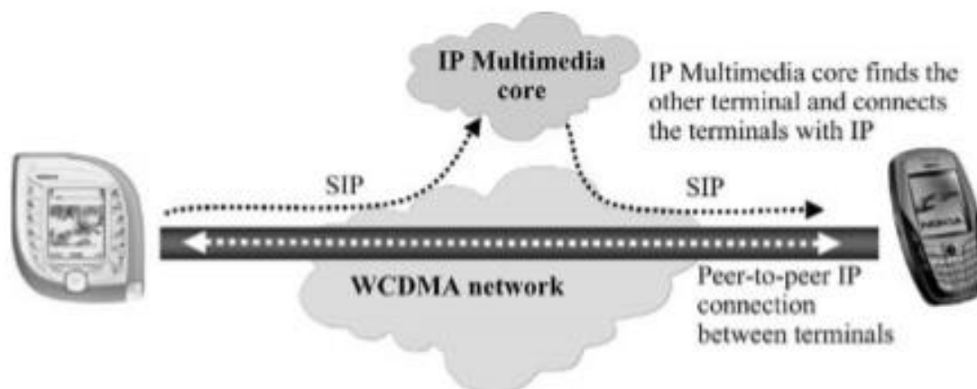
Slika 4. Osnovni princip IMS komponente, [1]
