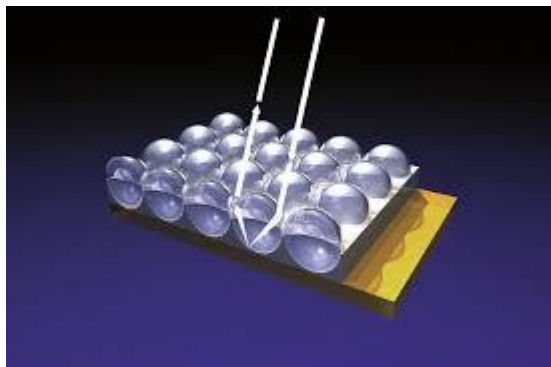
Slika 8. Sferična retrorefleksija
