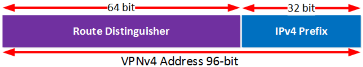
Slika 20. VPNv4 adresa
