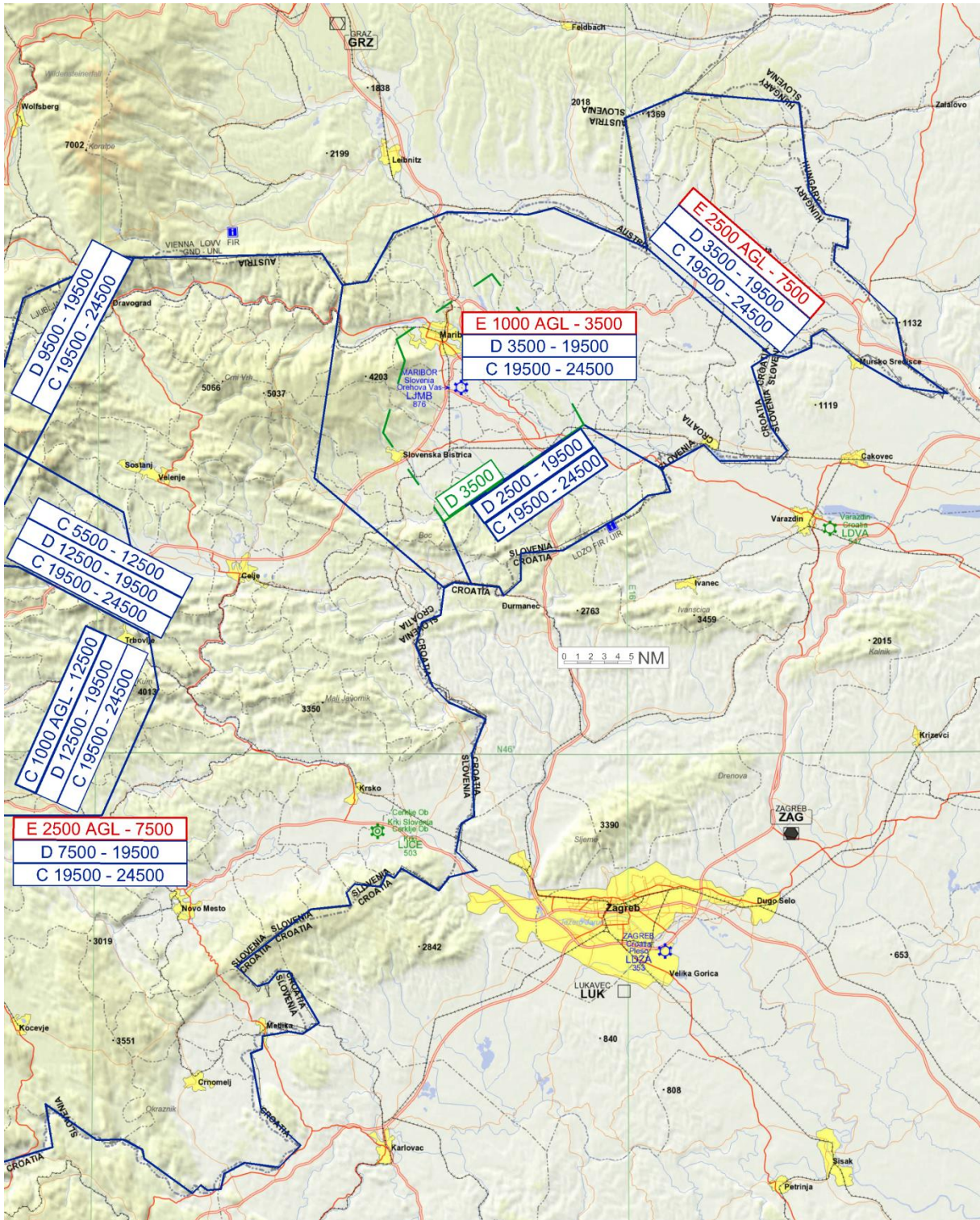
Slika 7. Struktura klasifikacije zračnog prostora oko aerodroma istočne Slovenije
