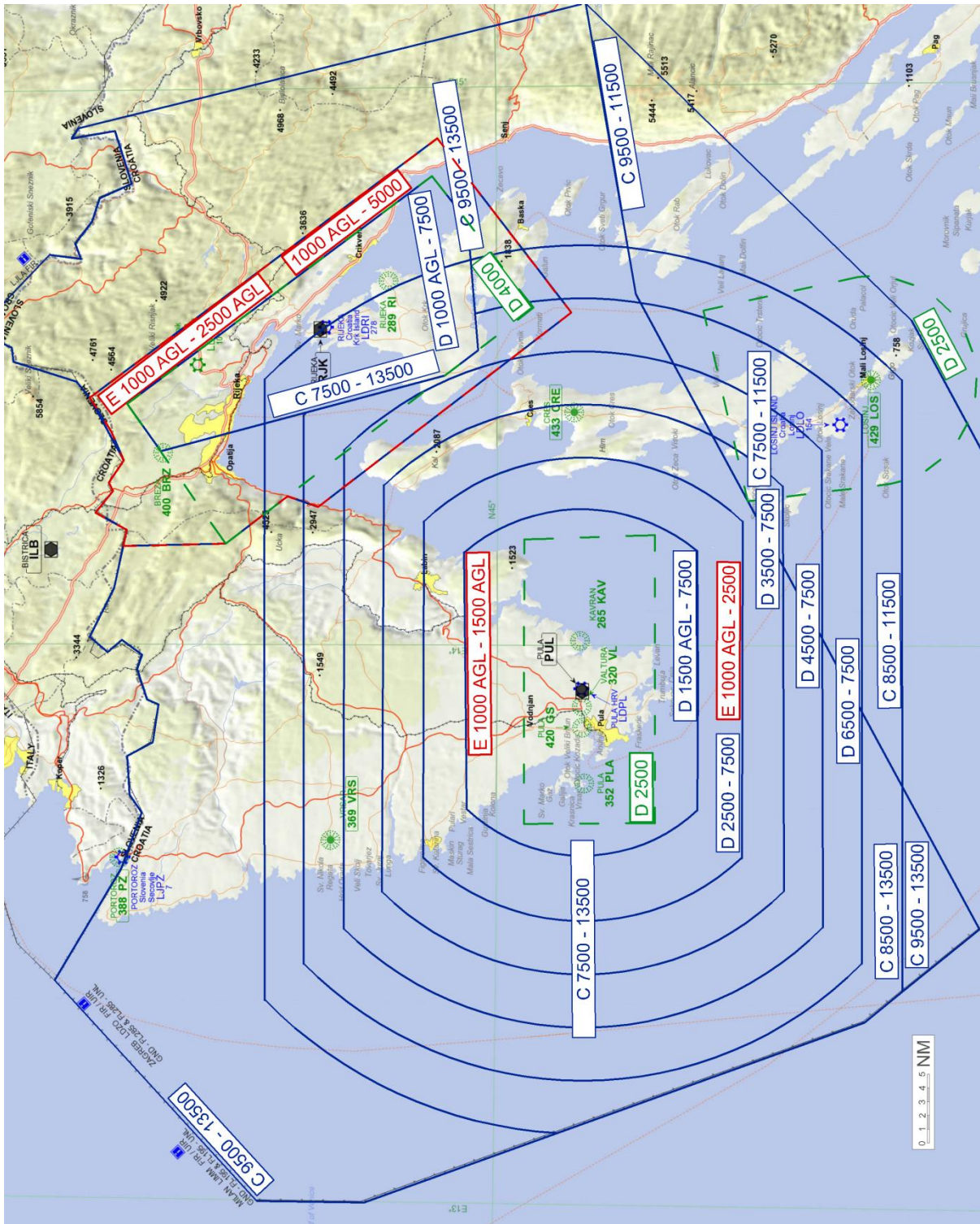
Slika 13. Prijedlog restrukturiranja zračnog prostora oko aerodroma sjevernog Jadrana
