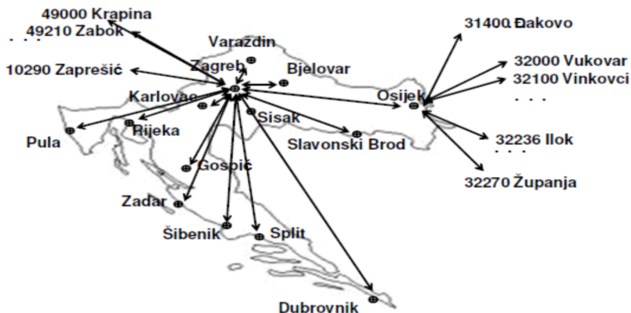
Slika 6.6. Prometni tokovi pošiljaka i razmjena zaključaka [7]
