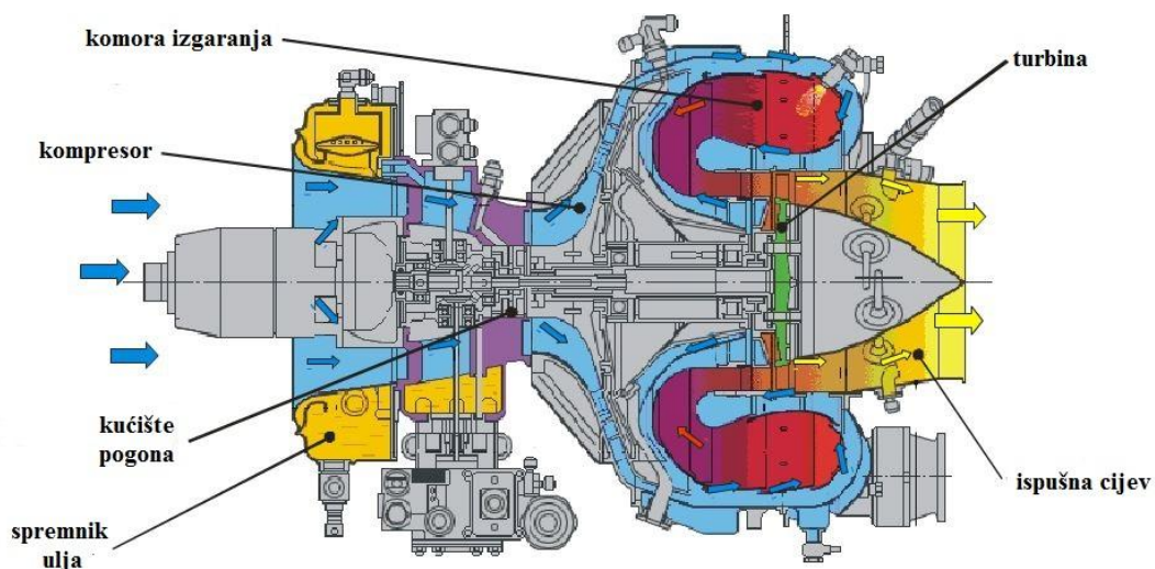
Slika 14. Ai-9V starter-generator [17]
