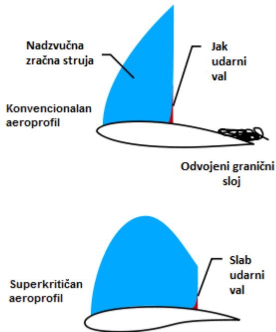
Slika 25: Konvencionalan i superkričan aeroprofil [7]
