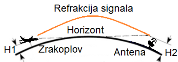
Slika 7. Utjecaj visine zrakoplova i refrakcija signala
