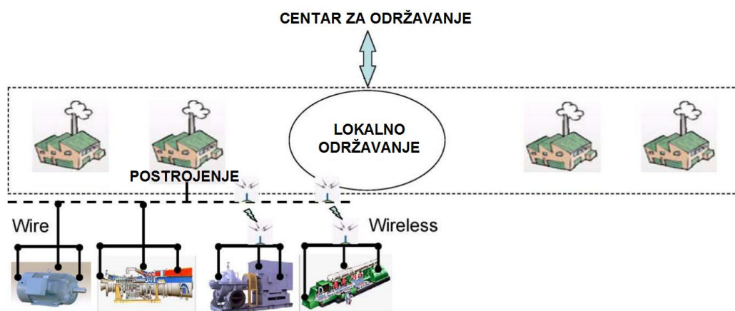
Slika 4.4. Arhitektura sustava E-održavanja, [3].
