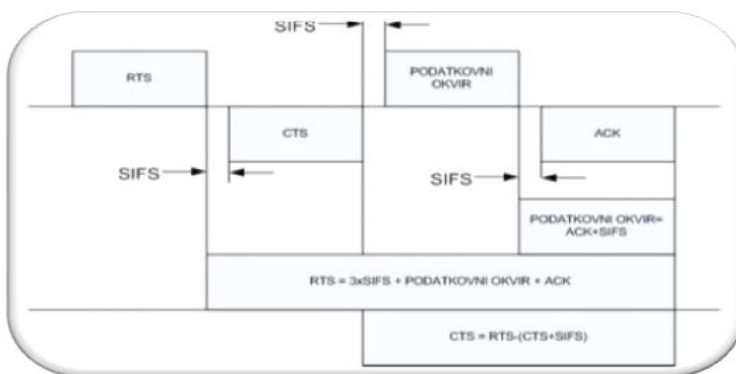
Slika 9. RTS/CTS mehanizam 26
