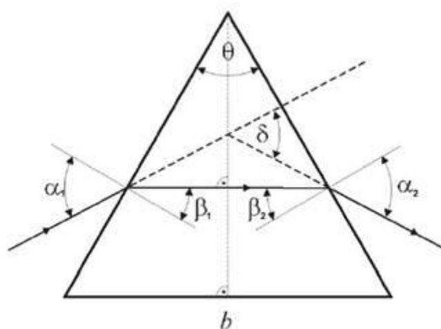
Slika 13. Lom svjetlosti kroz optičku prizmu [1]
