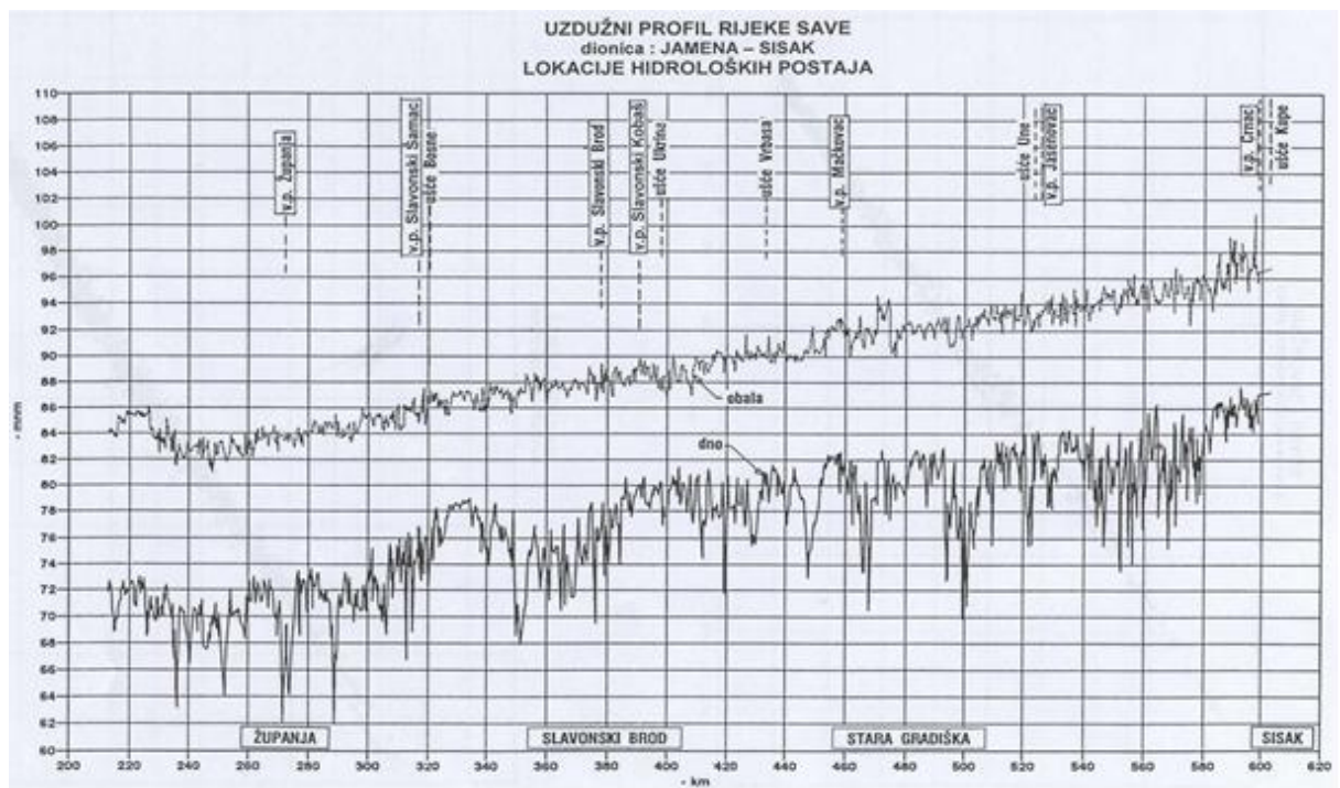
Slika 2. Longitudinalni profil, [7]
