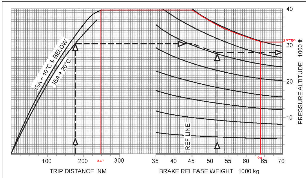
Slika 7. Optimalna visina leta za odabranu rutu
