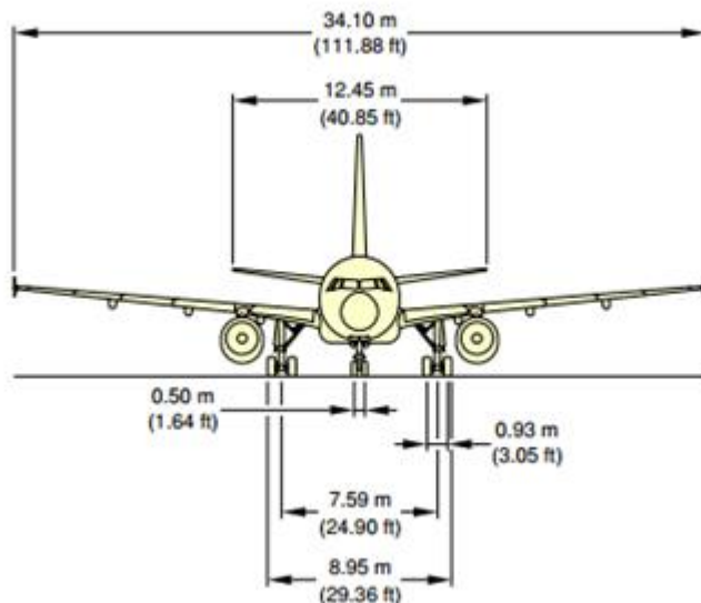
Slika 3. Dimenzije zrakoplova Airbus A320 prikazane iz nacrtna projekcije
