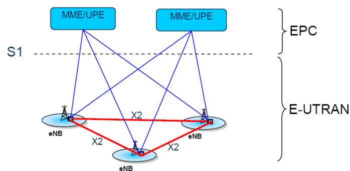
Slika 3.22. EPS arhitektura, [26]
