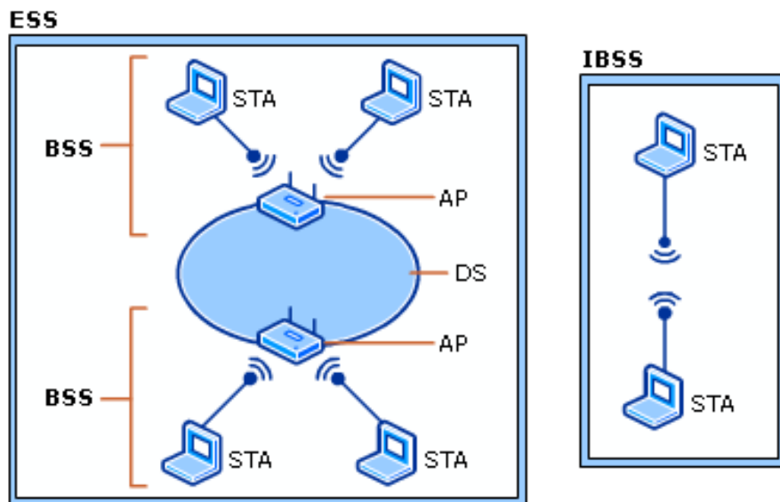
Slika 3.12. 802.11 arhitektura, [34]
