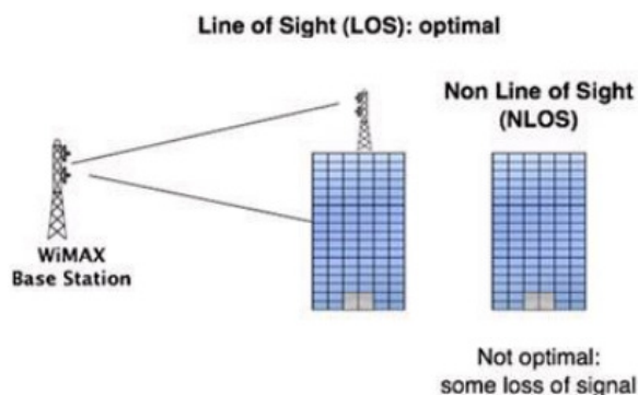
Slika 3.21. WiMAX optimalnost, [36]
