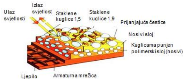
Slika 19. Sastav traka za privremene oznake na kolniku
