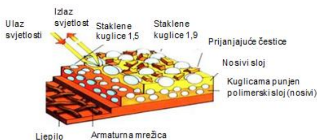
Slika 19. Sastav traka za privremene oznake na kolniku
