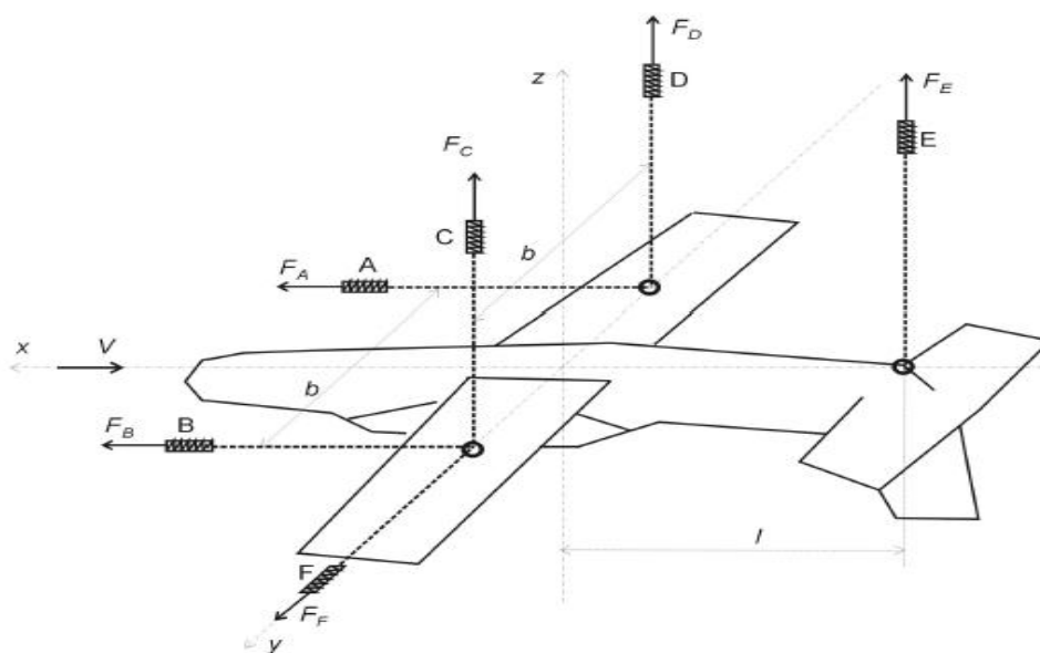
Slika 24 Žičana vaga
