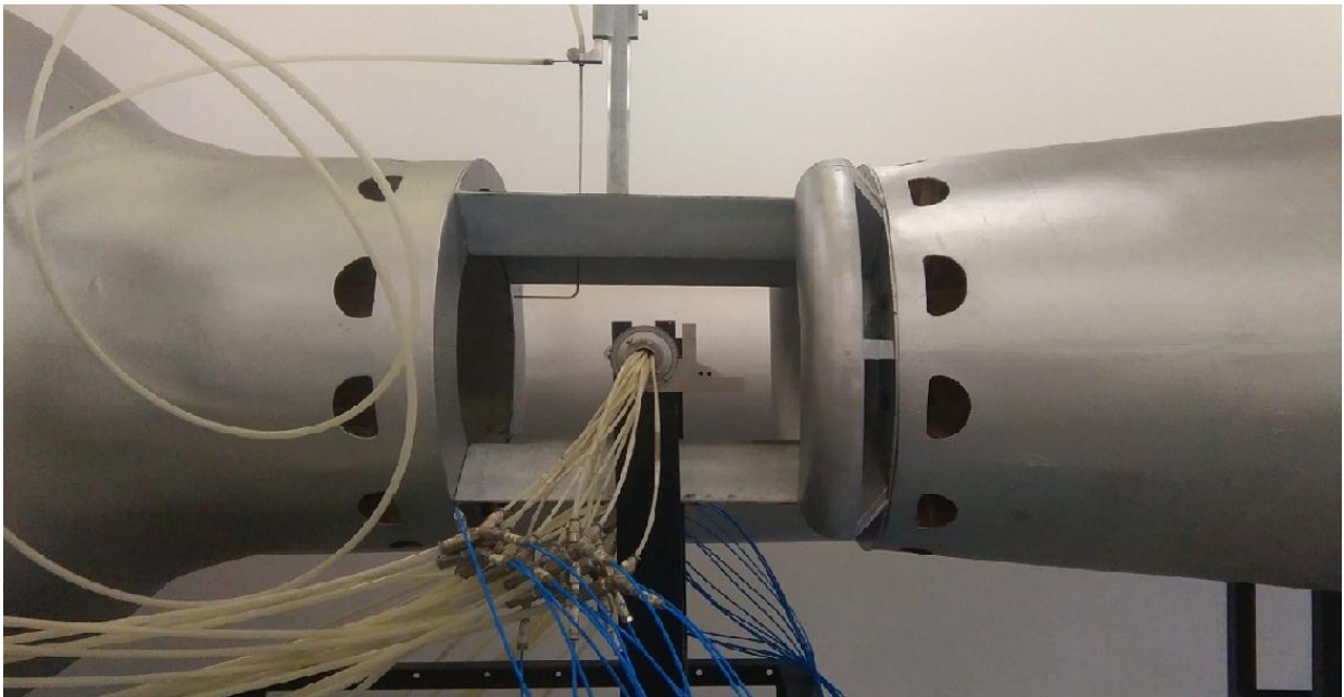
Slika 4. Ispitna sekcija
