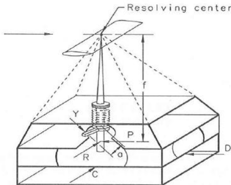
Slika 27. Piramidna vaga
