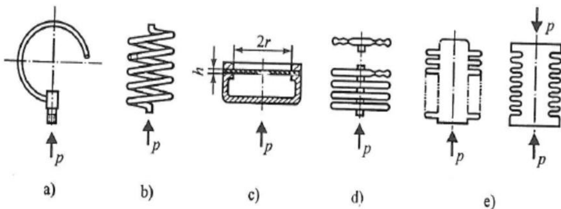
slika 14. Mehanički mjerni pretvornici tlaka
