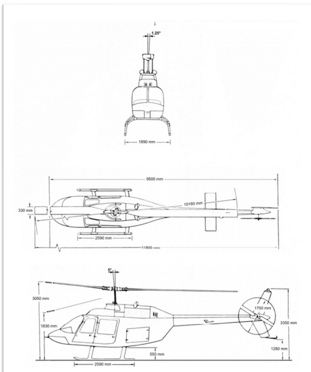
Slika 9. Dimenzije helikoptera
