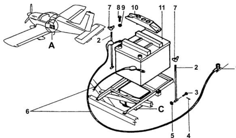
A – pozicija ugradnje glavne baterije, C – pozicija ugradnje pomoćne baterije 1 – spoj s konstrukcijom aviona, 2 – upornica, 3 – svornjak, 4 – rascjepka, 5 – podložna pločica (šajba), 6 – kablaza, 7 – matica, 8 – vijak pričvršćenja minus-pola, 9 – podložna pločica (šajba), 10 – držač baterije, 11 – glavna baterija CONCORDE RG 24-20
