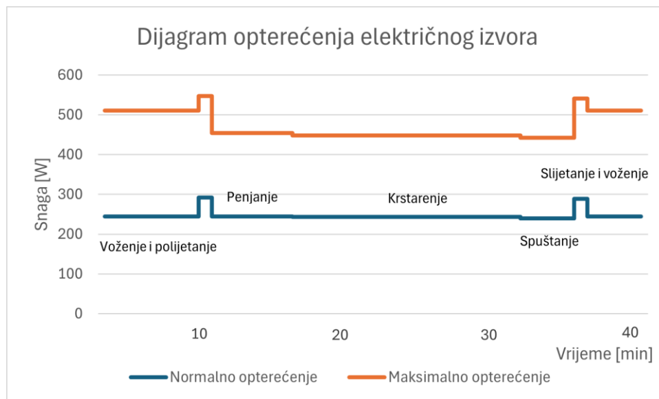
Slika 18. Elektroenergetska bilanca zrakoplova Zlin 242L
