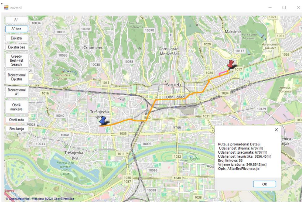
Slika 64. Detalji i ruta pronađena A* algoritmom bez Fibonaccijeve hrpe
