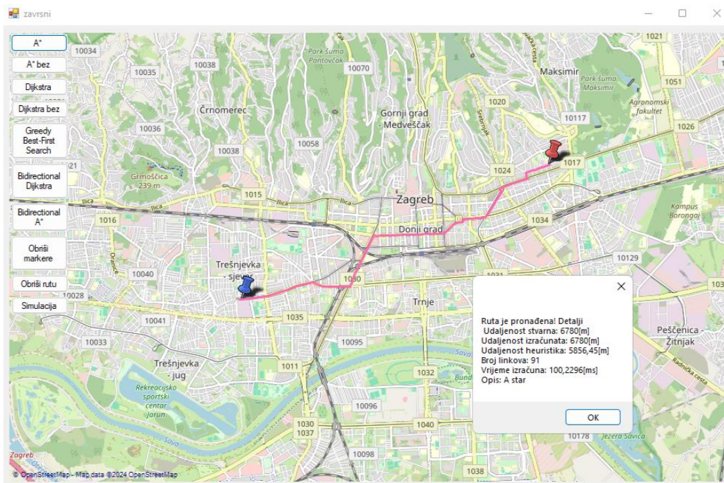
Slika 63. Detalji i ruta pronađena A* algoritmom
