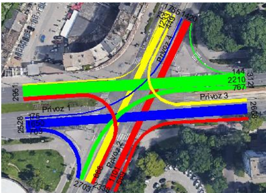
Slika 48. Grafički prikaz popodnevno vršnog opterećenja na raskrižju Savska cesta – Vukovarska ulica
