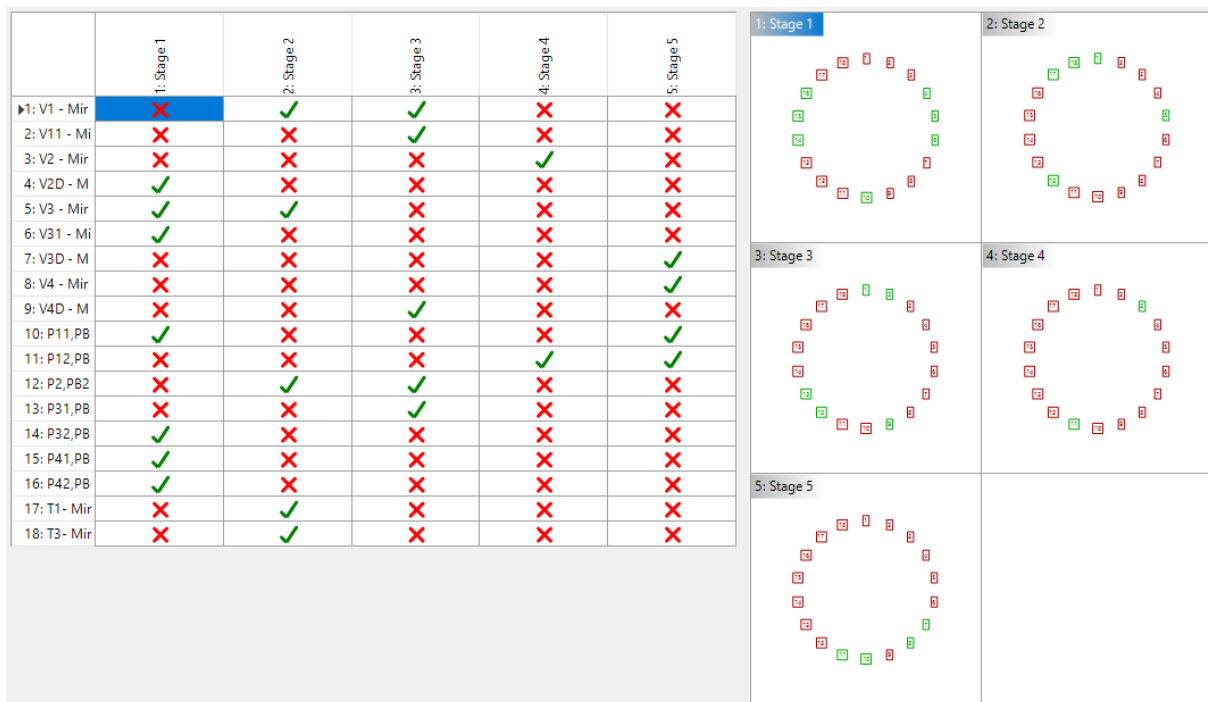
Slika 24. Prikaz rasporeda faza i pripadajućih signalnih grupa na raskrižju Miramarska cesta – Vukovarska ulica
