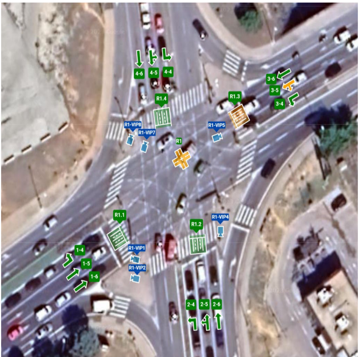
Slika 35. Plan postavljanja VIP uređaja Izvor: [autor]
