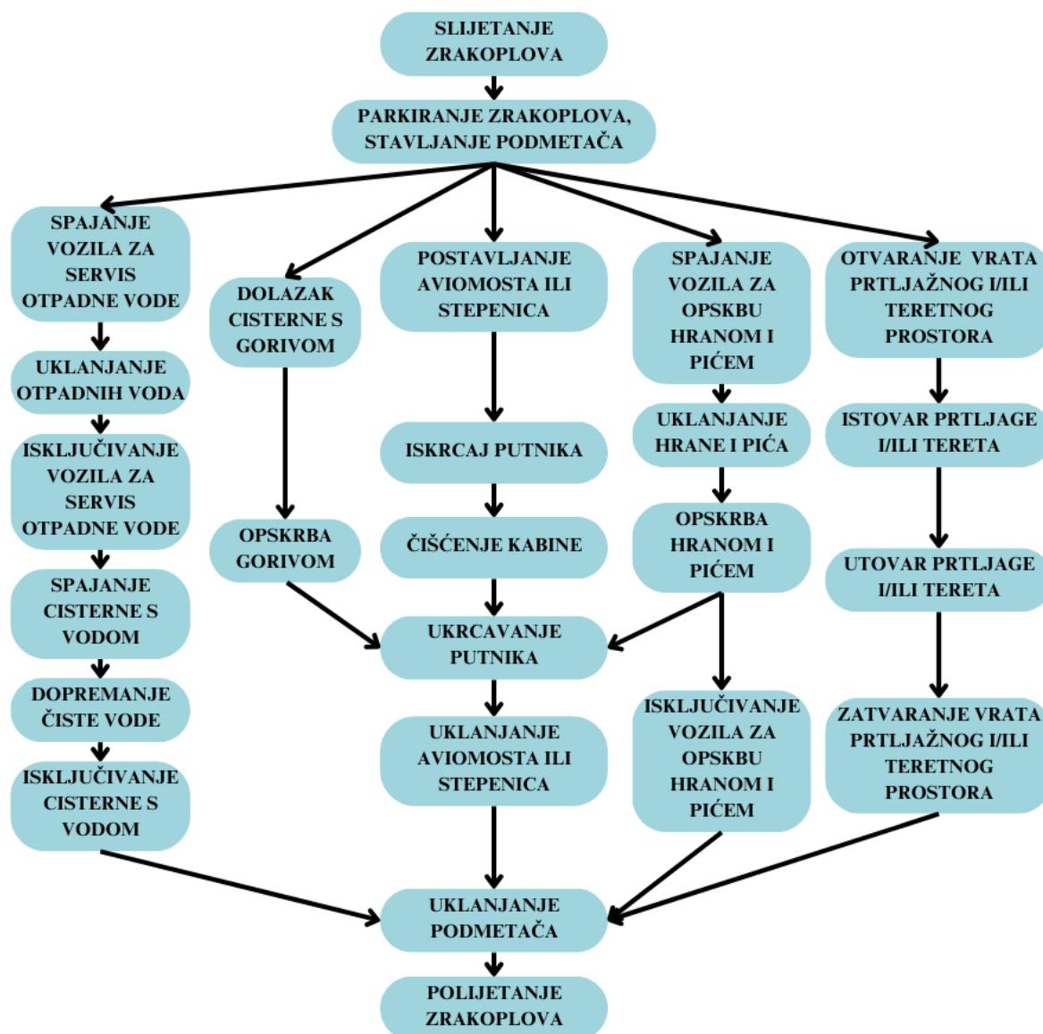
Slika 7. Prikaz sheme dijela procesa u zračnim lukama koji se odnose na prihvat i otpremu zrakoplova.
