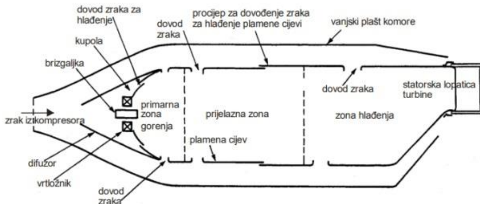
Slika 1 Konvencionalna komora izgaranja [5]
