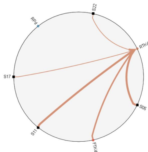
Slika 32: Izlazni rezultati IBM SPSS Statistics za provedeni TCM – prikazi uzročnih veza za ostvarene tonske kilometre u domaćem prometu gdje S24 nije uključen u model
