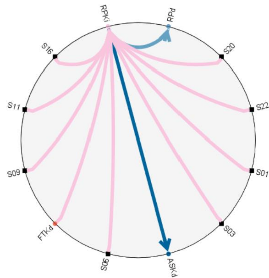
Slika 30: Izlazni rezultati IBM SPSS Statistics za provedeni TCM – prikazi uzročnih veza za ostvarene putničke kilometre u domaćem prometu gdje S24 nije uključen u model
