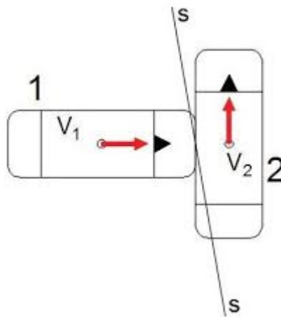
Slika 3 Bočni sudar
