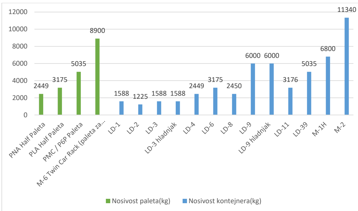
Grafikon 2. Graf pojedinačne nosivosti transportnih jedinica za zračni prijevoz
