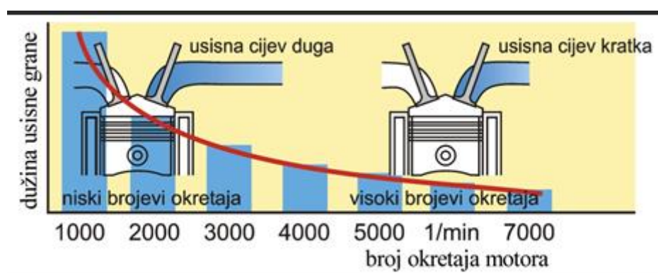
Slika 11 prikaz ovisnosti duljine usisne cijevi i broja okretaja motora, [1]
