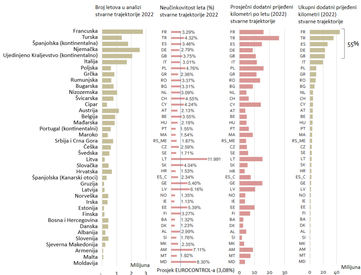
Slika 40. Horizontalna en-route neučinkovitost stvarnih putanja po državama u 2022. godini [29].
