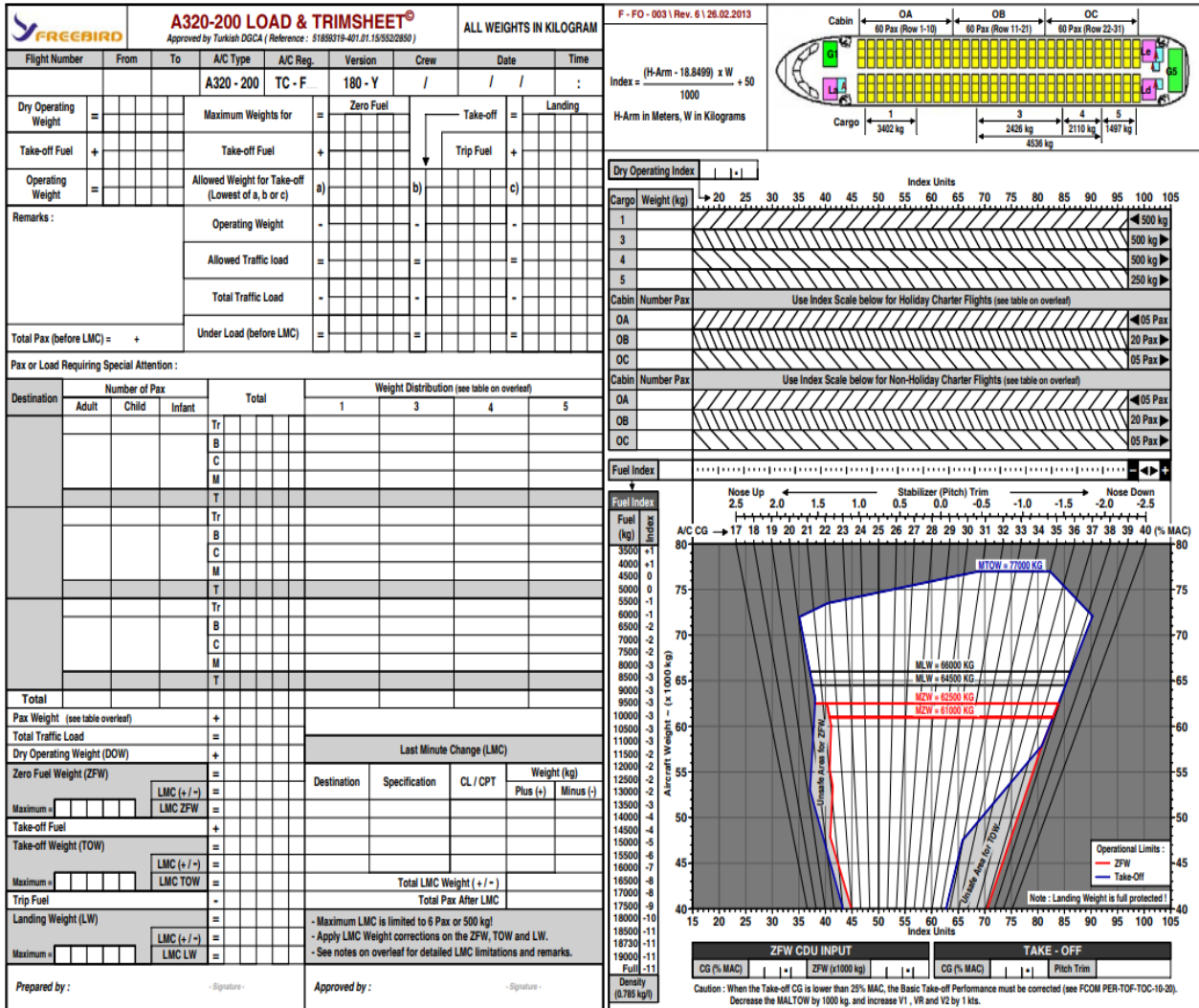
Slika 15. Prazna lista opterećenja i uravnoteženja za zrakoplov A320-200 kompanije Freebird Airlines Izvor [19]
